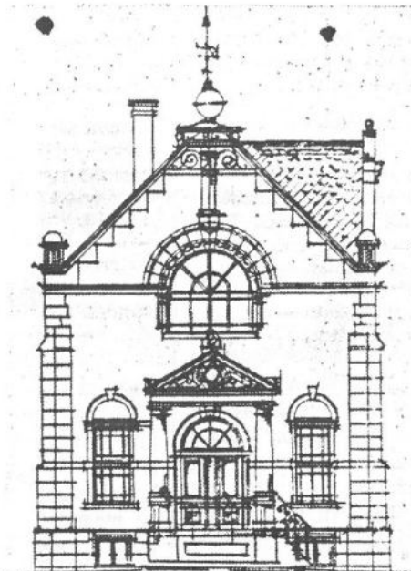
Das ist der Aufriß der Vorderseite der Synagoge in Nastätten, die 1902-04 an der Ecke Brühl-/Rheinstraße errichtet und 1938 zerstört wurde.
